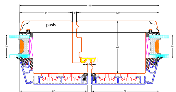
L1: Lodpost lodret indadgående dør
