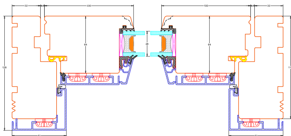
D1: Sidekarme døre, indadgående
