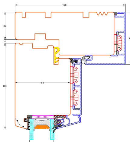
D2: Topkarme døre, indadgående
