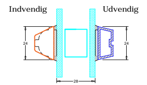
D3: Dørtrin indadgående dør (kan leveres med dobbelt spændestykke)
