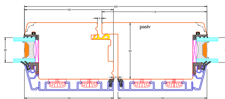
L1: Lodpost lodret udadgående dør
