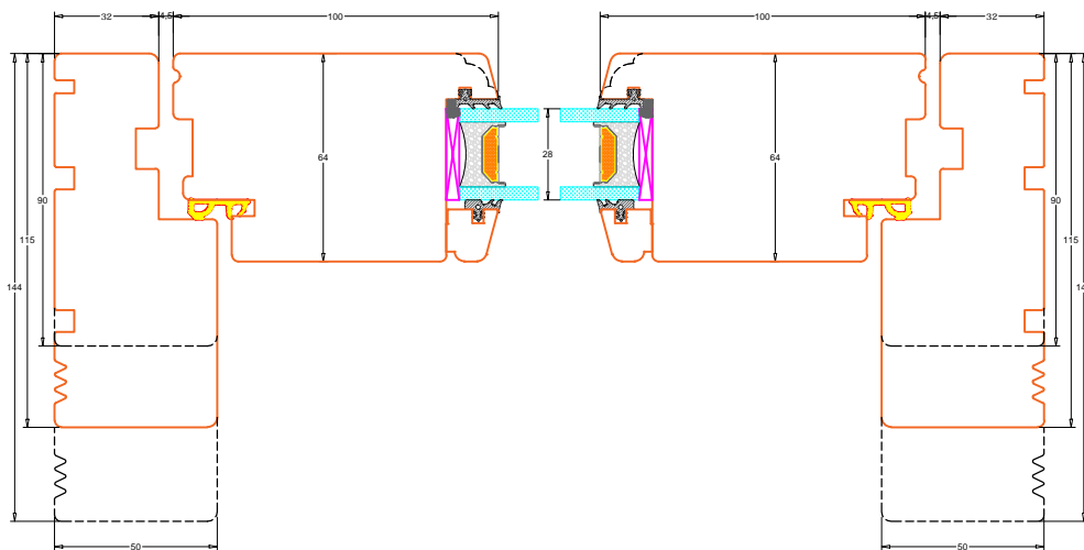
D1: Sidekarme døre, indadgående
