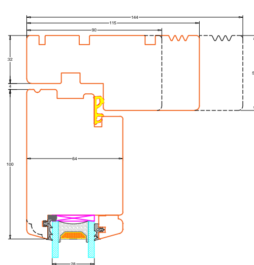
D2: Topkarme døre, indadgående
