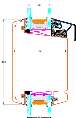
L2: Lodpost vandret
