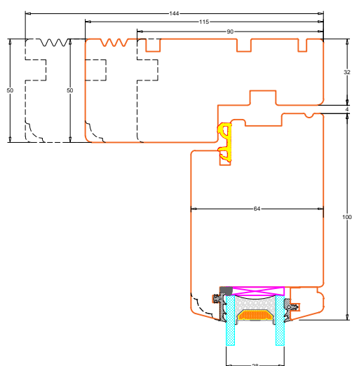
D2: Topkarme døre, udadgående
